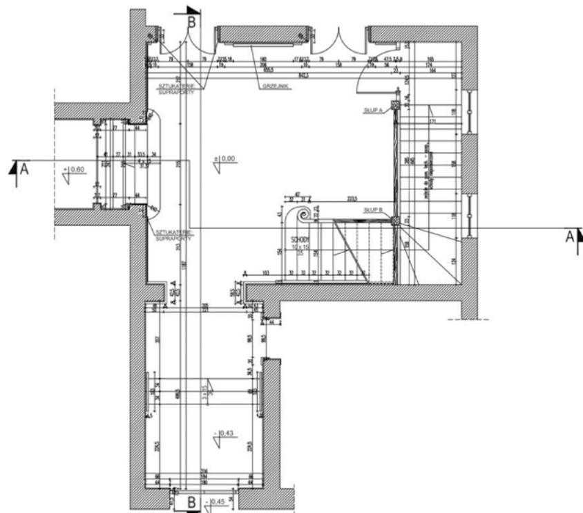
Fragment inwentaryzacji budynku Rektoratu Politechniki Poznańskiej, pl. M. Skłodowskiej-Curie 5, inwentaryzacja 2011, prowadzący: prof. dr inż. arch. T. Bardzińska-Bonenberg, wykonali: S. Menzel, P. Michałak, J. Walczak, S. Wędrychowicz, M. Zajda
